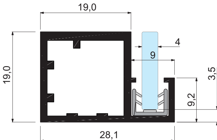
Tehnički detalji profila za izradu fronta
